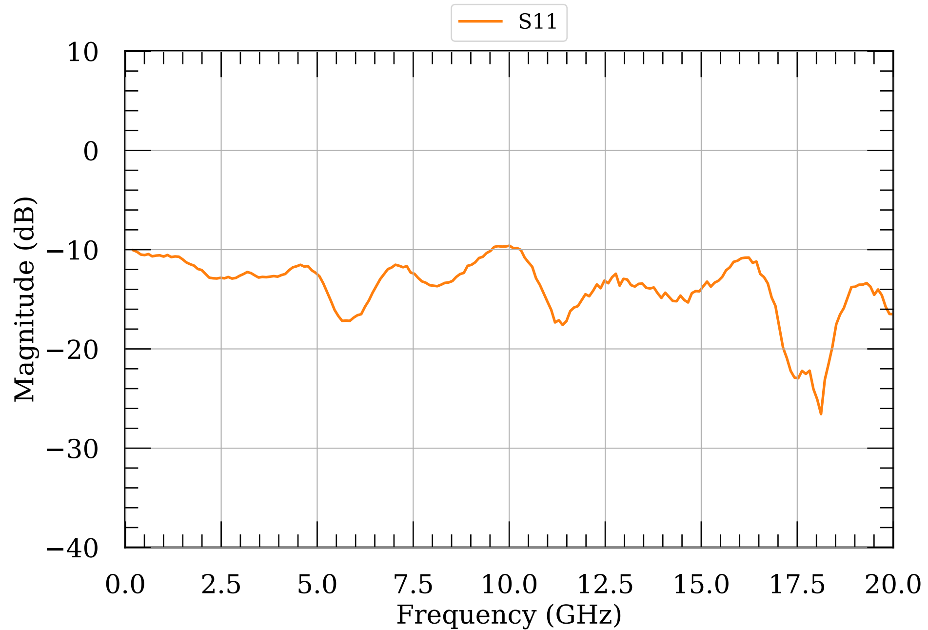
LNA S-params module015v2
